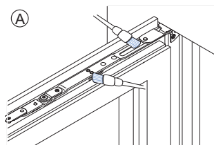
Bild 1: Schere (Flügel)
